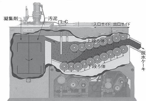
ヘリオス脱水機構造
