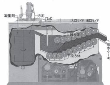
ヘリオス脱水機構造
